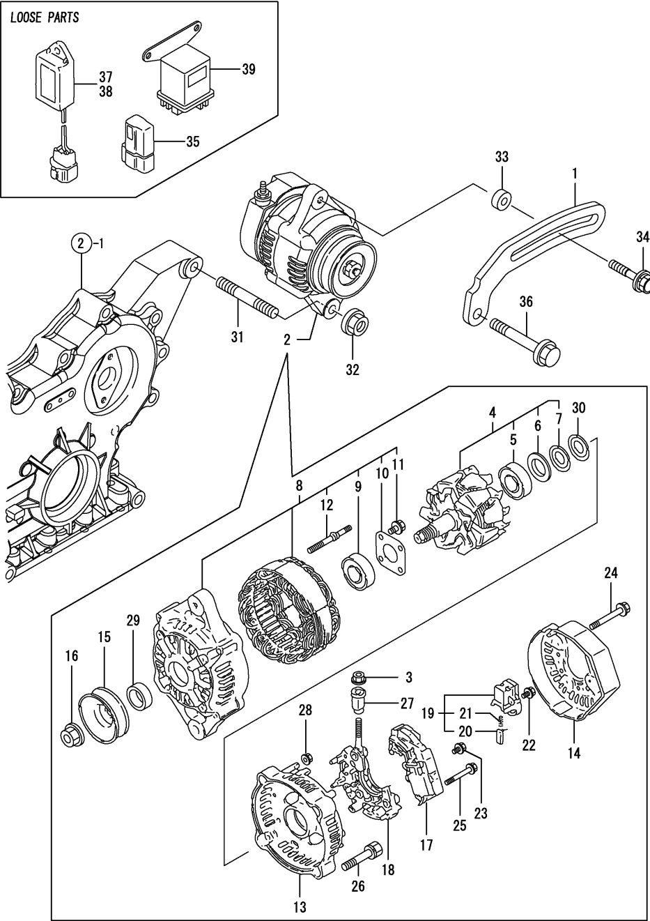
OCV10-G97100 Fig.15.GENERATOR
