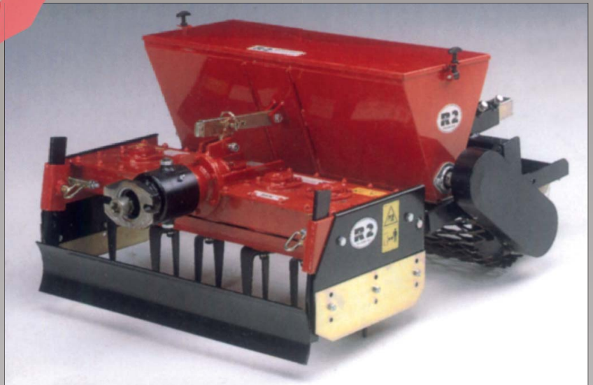
Rotorharve med gittertromle og såmaskine. Arbejdsbredde 75 cm.
