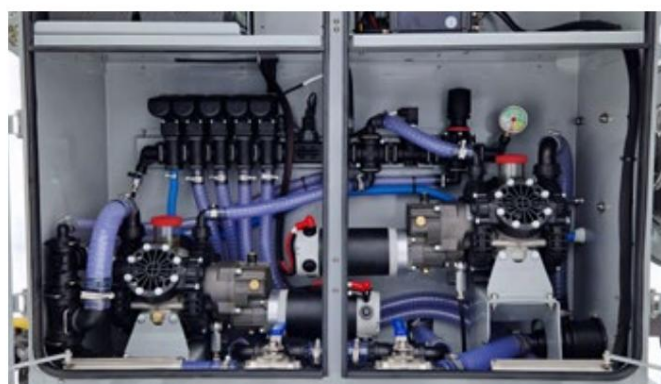
Selvansugende højtryks- og flowmembranpumper, motorer og ventiler i lukket kabinet
