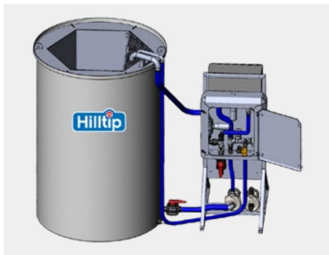
Blandetank og styreskab
