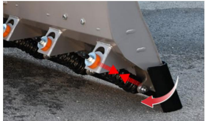
Skærende kant med udløserfjedere
