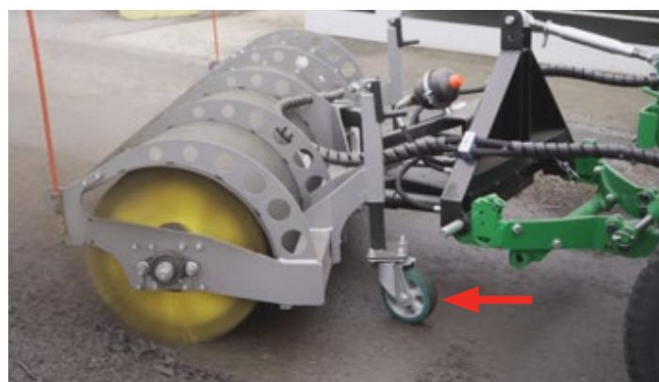
Støtthjul
